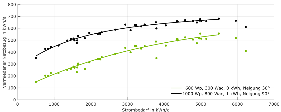
Abbildung 5 Beispielhafte Regressionsanalyse des Autarkiegrads in Abhängigkeit von der PV-Generatorleistung, der Speicherkapazität und der Neigung der Systemkonfiguration bei einer südlichen Ausrichtung.
