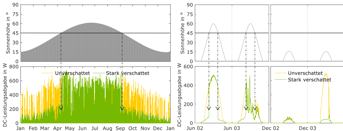
Abbildung 3 Gegenüberstellung der Sonnenhöhe und DC-Leistungsabgabe des PV-Generators (600 Wp) im unverschatteten und stark verschatteten Fall.
